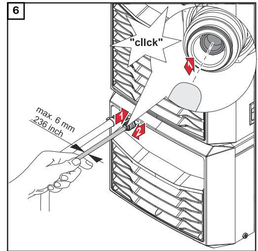
Pritisnite brtveni stožac u priključku za predtok rashladnog sredstva prema nazad
