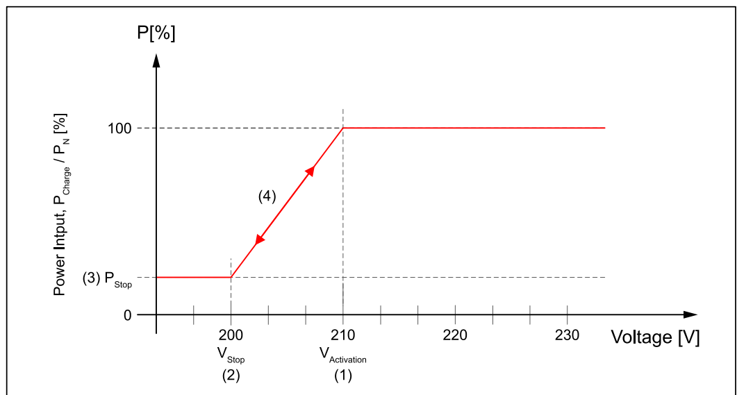
Ladeleistungsbegrenzung bei Überschreiten von Activation Threshold Undervoltage .
